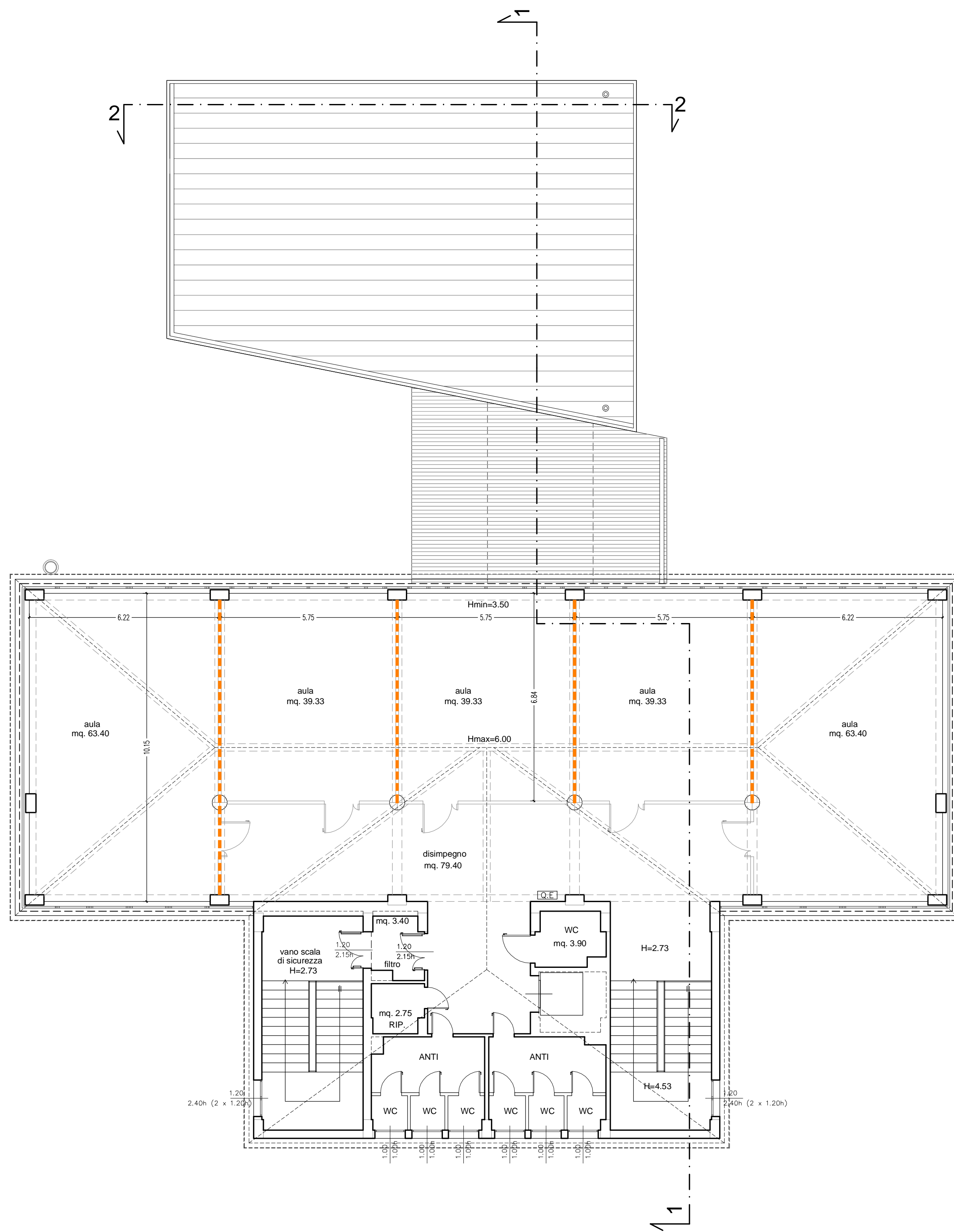
PIANO SECONDO - SCALA 1:100
