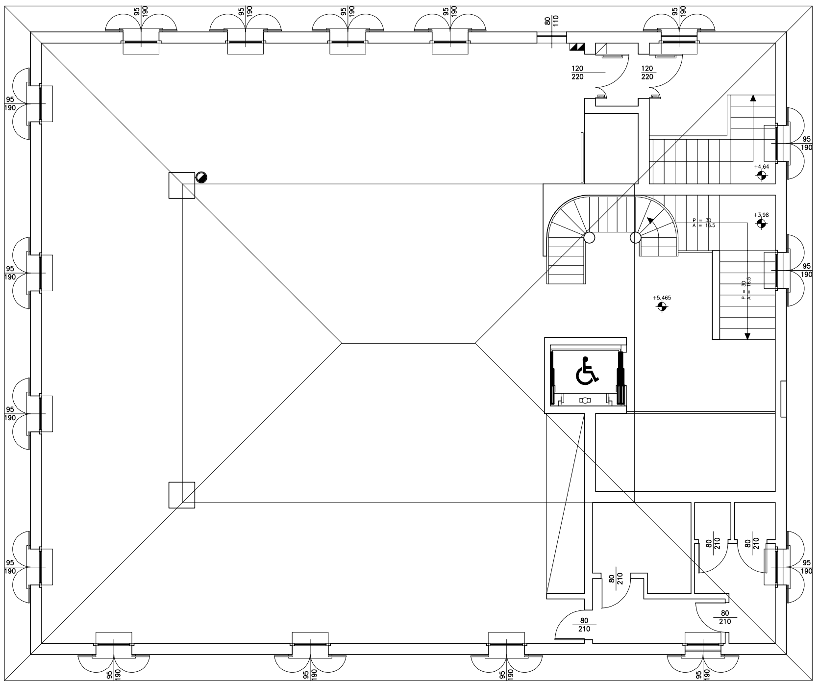
PIANO PRIMO Scala 1:50
