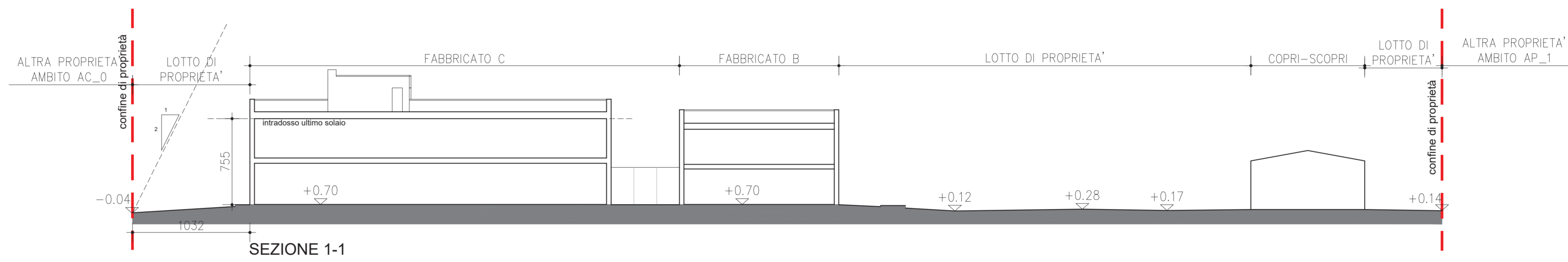
SEZIONE 1-1
