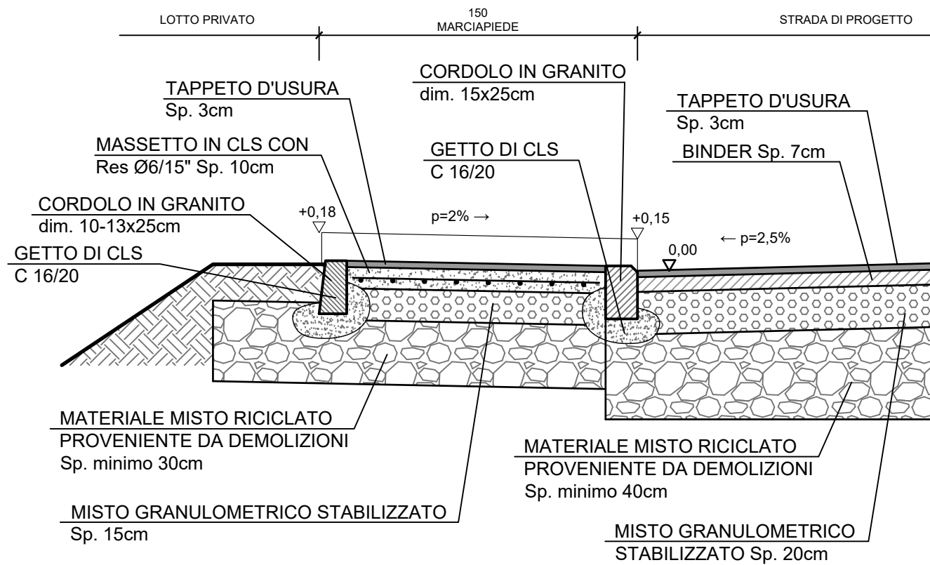
SEZIONE A-A 1:25
