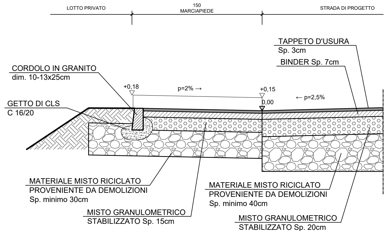
SEZIONE B-B 1:25
