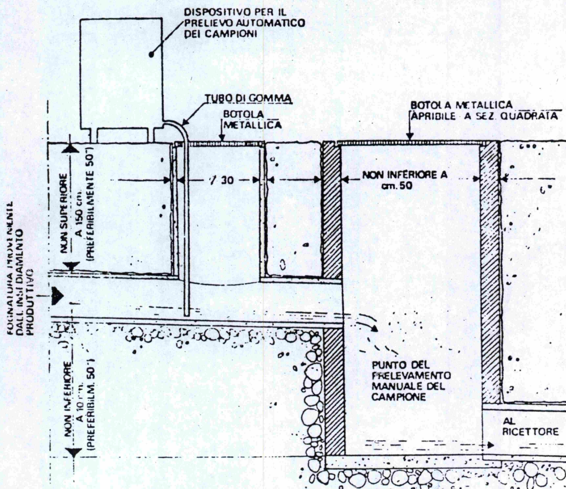
SEZIONE SCHEMA POZZETTO DI PRELEVAMENTO
