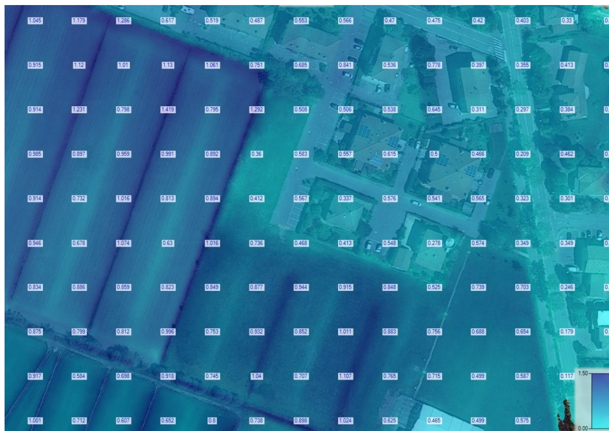
Figura 18 – Rappresentazione del dettaglio dell'esondazione in corrispondenza del sito di interesse con l'indicazione dei valori di altezza d'acqua raggiunta.
